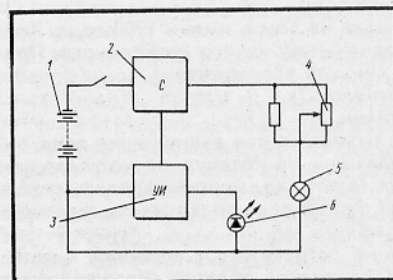
РИС. 2. ФУНКЦИОНАЛЬНАЯ СХЕМА ЭКСПОНЕТРА: 1 — ИСТОЧНИК ПИТАНИЯ; 2 — СТАБИЛИЗАТОР НАПРЯЖЕНИЯ; 3 — УСТРОЙСТВО ИНДИКАЦИИ РАЗРЯДА БАТАРЕИ; 4 — ПЕРЕМЕННЫЙ РЕЗИСТОР; 5 — ЛАМПА НАКАЛИВАНИЯ; 6 — СВЕТОДИОД
